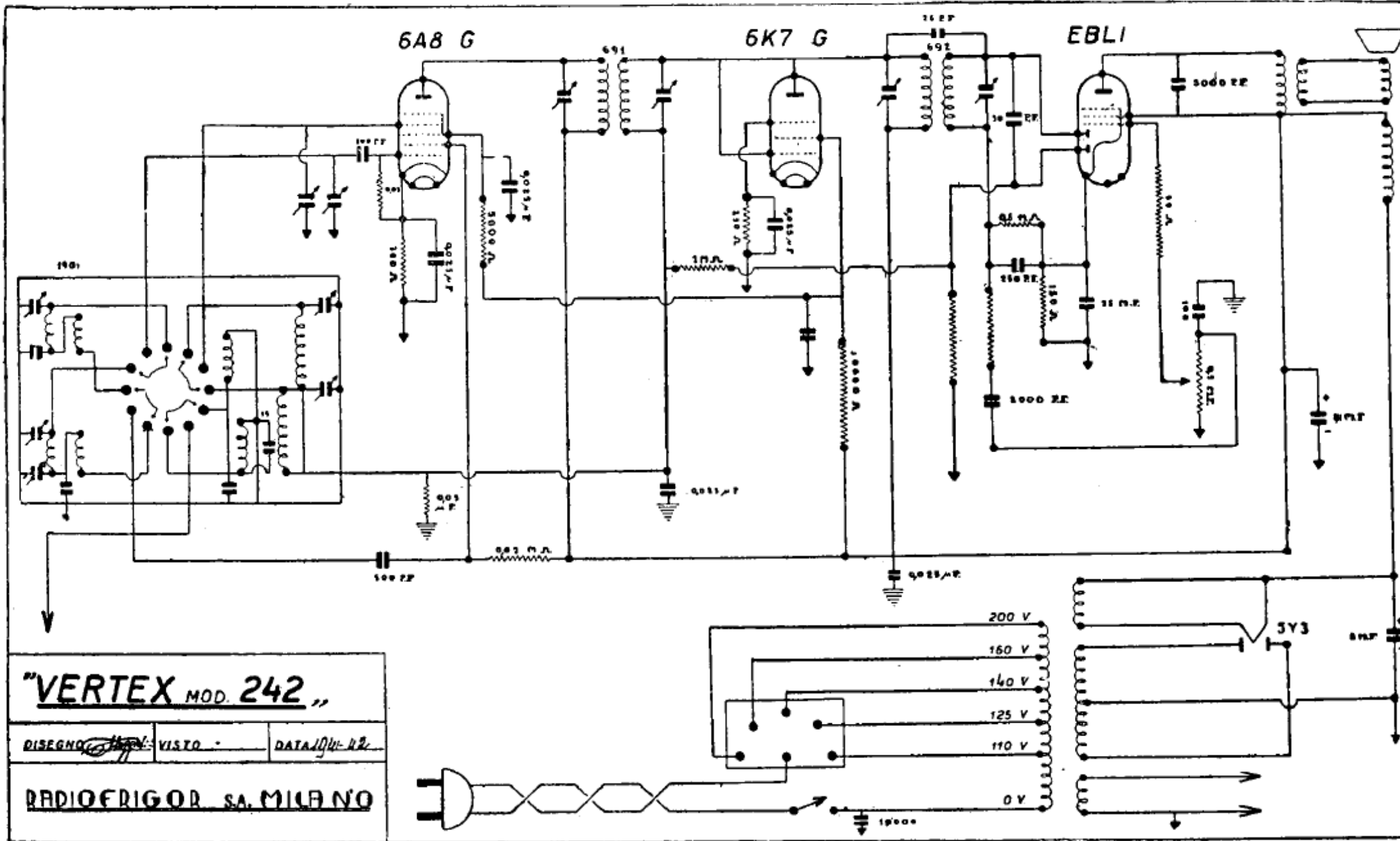
VERTEX (S. A. RADIOFRIGOR). — Mod. «242 e 421 con 6AY8». — Produzione 1941-1942. — Media frequenza: 467 kHz. — Onde medie e corte. — Avvolgimento di campo: 2500 ohm.
